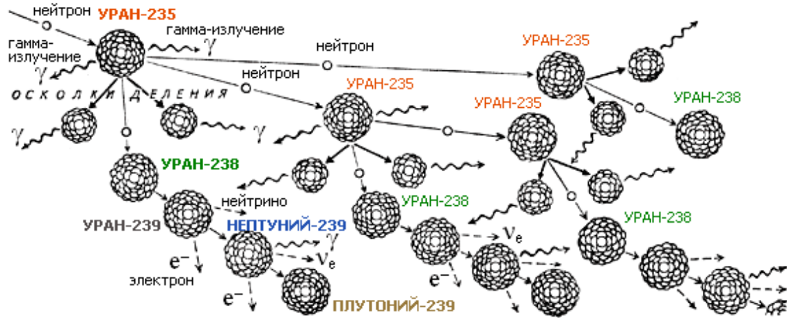
Рис. 18. Схема образования плутония-239 при цепной реакции деления ^{235}\text{U}
