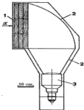
Черенковский счетчик: \chi – регистрируемая частица, 1 – радиатор, 2 – светопровод, 3 – ФЭУ.
