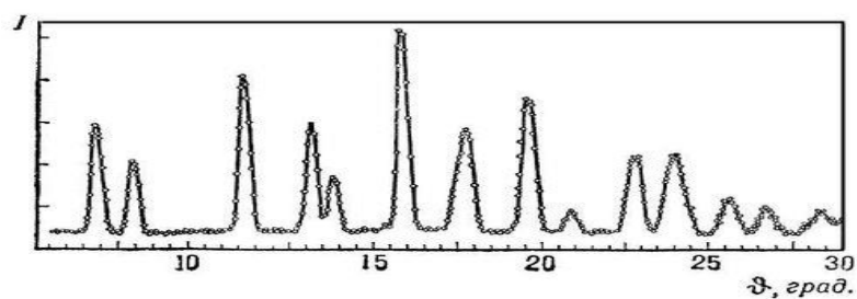
Нейтронограмма поликристаллического образца \text{BiFeO}_3
