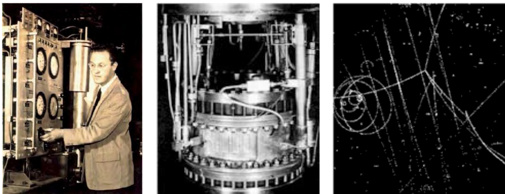
На снимках: А. Глезер у пульта управления его пузырьковой камерой, внешний вид камеры Глезера и фотография треков нескольких частиц, полученная в магнитном поле.
