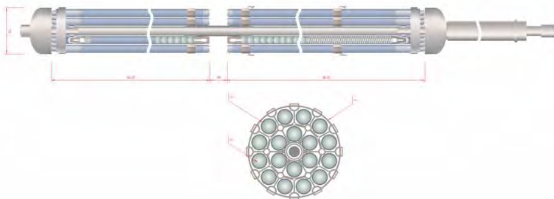
Тепловыделяющая сборка реактора РБМК
