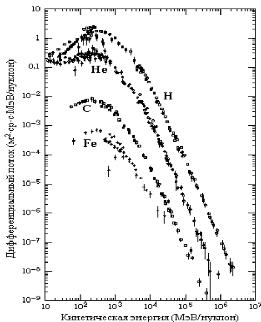
Рис. 15. Основные компоненты первичных космических лучей
