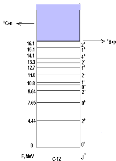
Структура энергетических уровней ядра ^{12}\text{C}
