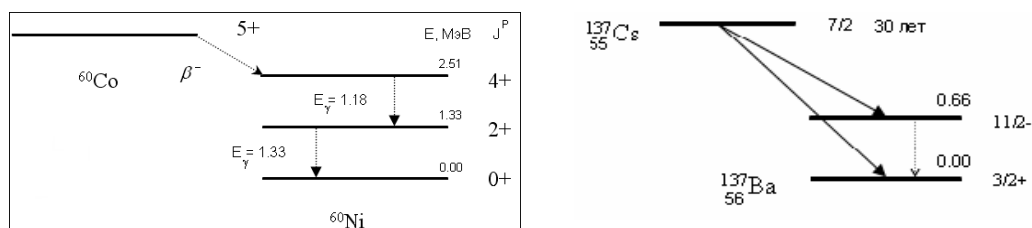
Структура некоторых уровней и энергетических переходов в ядрах ^{60}\text{Co} ( ^{60}\text{Ni} ) и ^{137}\text{Cs} ( ^{137}\text{Ba} )
