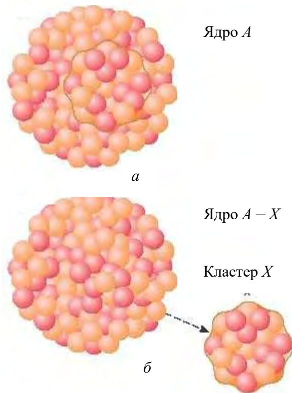
Рис. 1. Схема выхода кластера из атомного ядра: а – кластер X находится внутри ядра A ; б – кластер X вылетел из ядра
