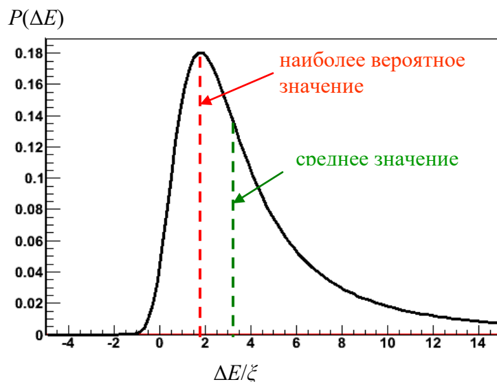
Распределение Ландау
