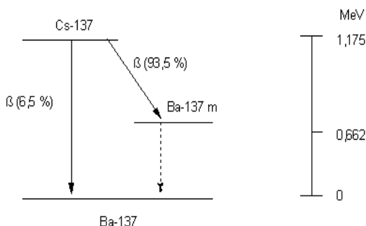
Рис. 10. Схема распада ^{137}\text{Cs}
