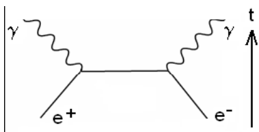
Аннигиляция электрона и позитрона с рождением пары фотонов
