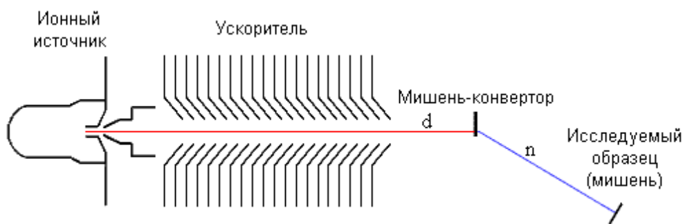
Схема нейтронного генератора
