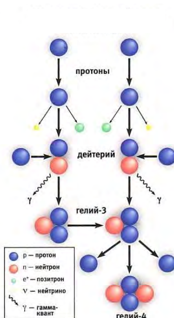
Рис. 12. Протон-протонный цикл синтеза гелия
