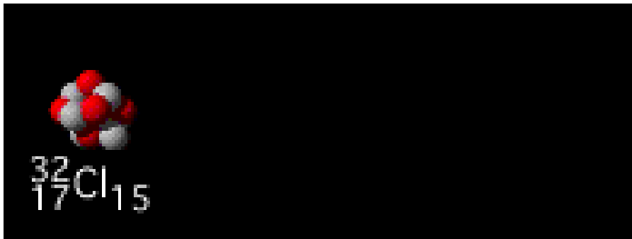
Рис. 5. Бета-распад изотопа ^{32}\text{Cl}
