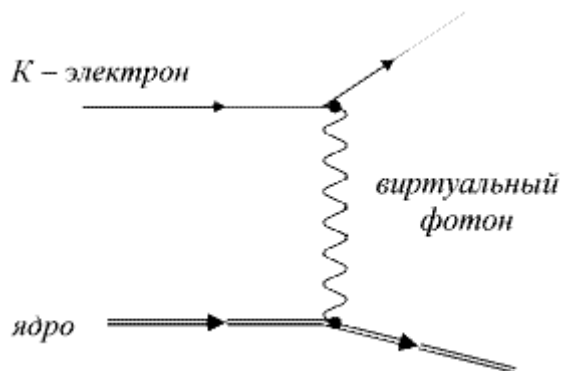
Рис. 7. Диаграмма Феймана для внутренней конверсии
