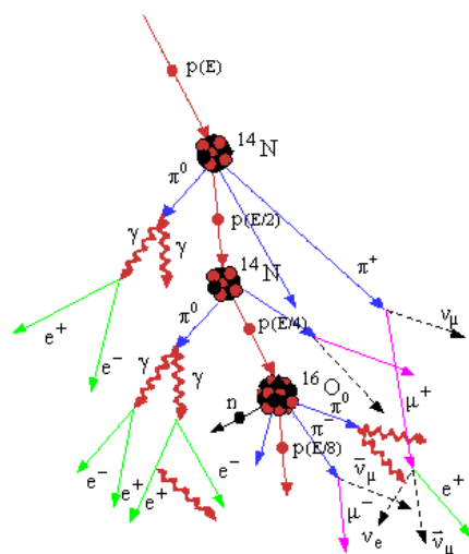
Рис. 16. Образование космического ливня протоном высокой энергии
