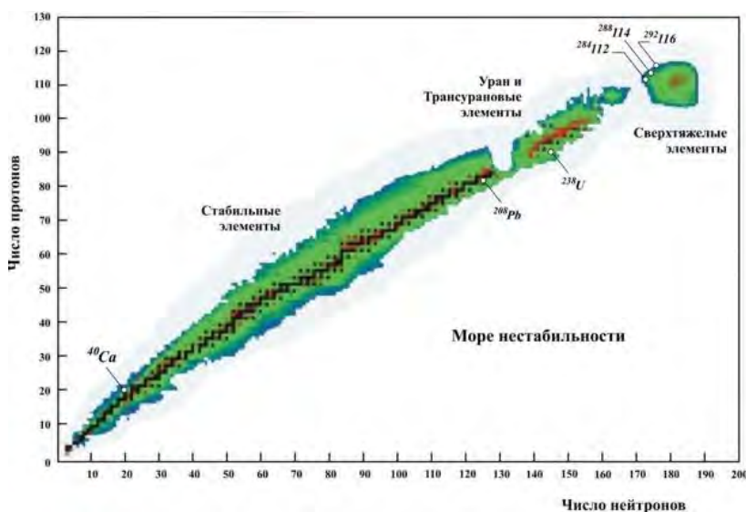
Рис. 9. Область стабильности изотопов
