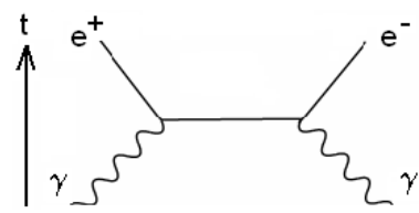
Эффект рождения пар при рассеянии фотона высокой энергии на атоме
