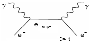
Диаграмма Фейнмана для рассеяния фотона на свободном электроне
