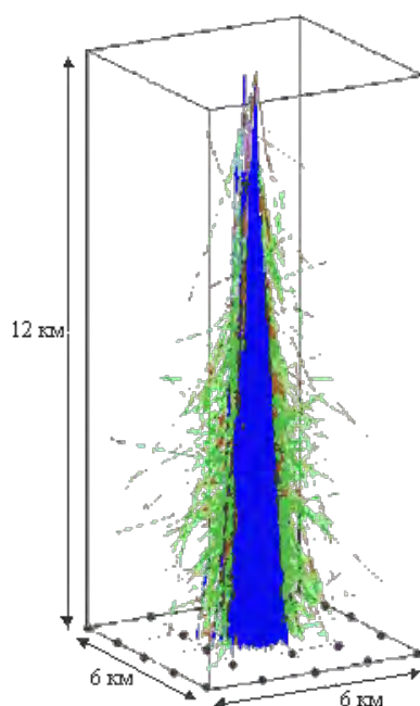
Рис. 17. Развитие широкого атмосферного ливня, инициированного космическим протоном
