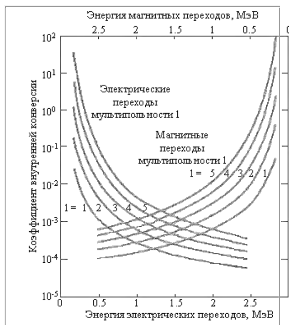
Рис. 8. Теоретически рассчитанные коэффициенты внутренней конверсии для атома циркония
