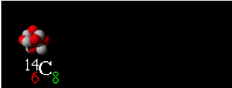
Рис. 4. Бета-распад изотопа ^{14}\text{C}
