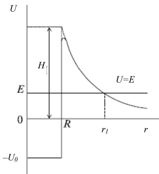
Рис 3. Потенциальная яма для альфа-частиц в ядре: U – потенциальная энергия, U_0 – основной уровень, H – высота барьера, r – расстояние от центра ядра, E – начальная энергия альфа-частицы, R – радиус ядра, r_1 – расстояние отрыва частицы от ядра
