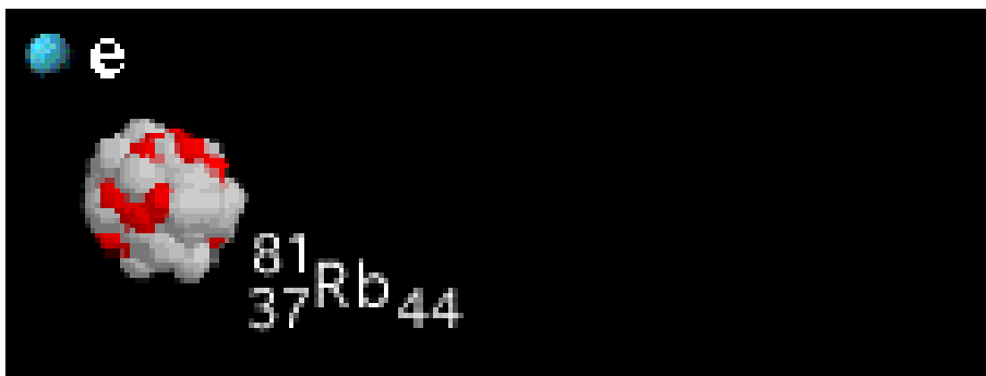
Рис. 6. Бета-распад изотопа ^{81}\text{Rb}
